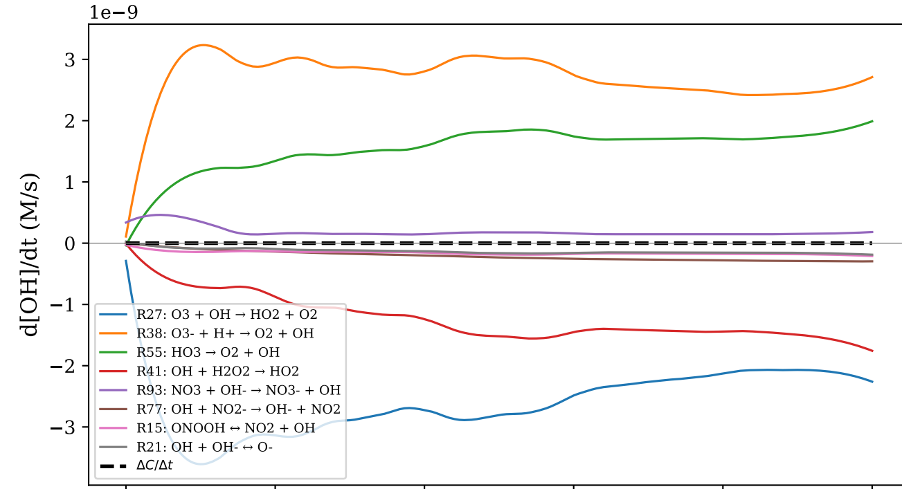
(d) H + [final=19.42 μM]
