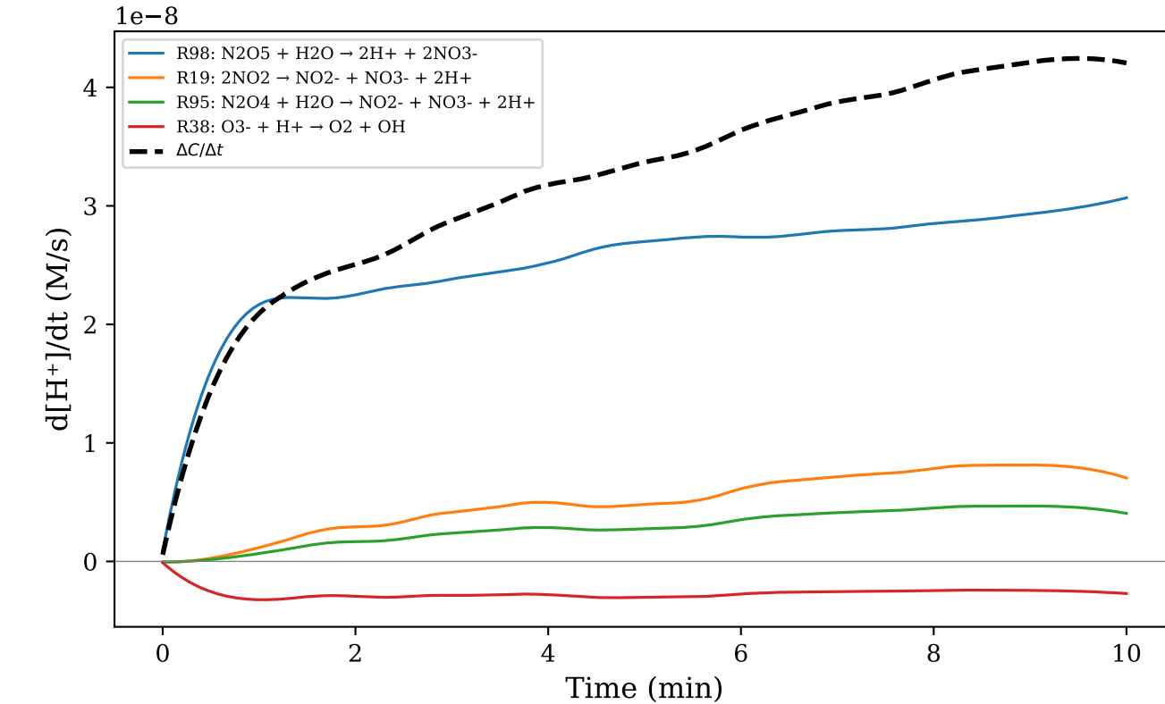
(d) H + [final=19.42 μM]
